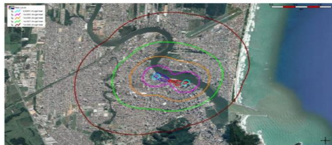
Figura 25 – Risco Individual das Instalações do Porto de Itajaí
