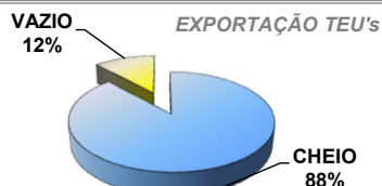
EXPORTAÇÃO TEU's
